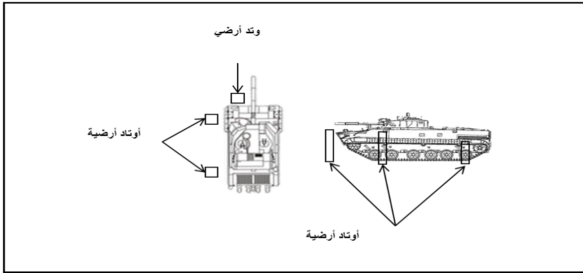
الشكل رقم (24) تأشير موقع ناقلة القتال المدرعة بالأوتاد الأرضية
