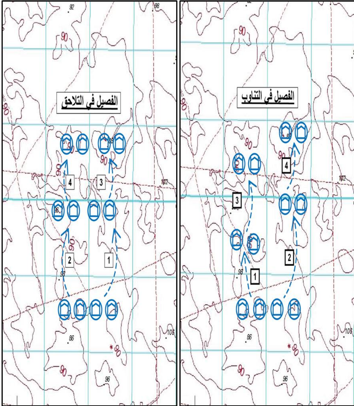
الشكل رقم (60) طريقة التلاحق والتناوب بالآليات
