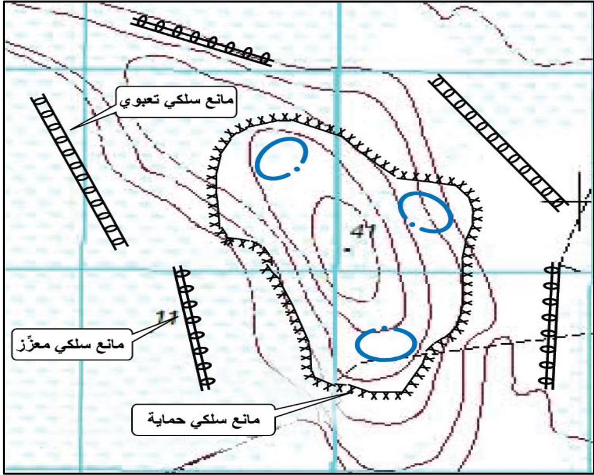
الشكل رقم (25) مثال على الأنواع الثلاثة من الموانع السلكية
