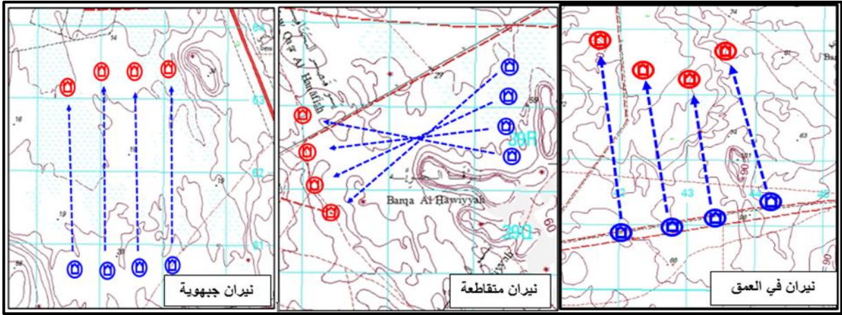
الشكل رقم (7) ثلاثة أنواع من أشكال الرماية
