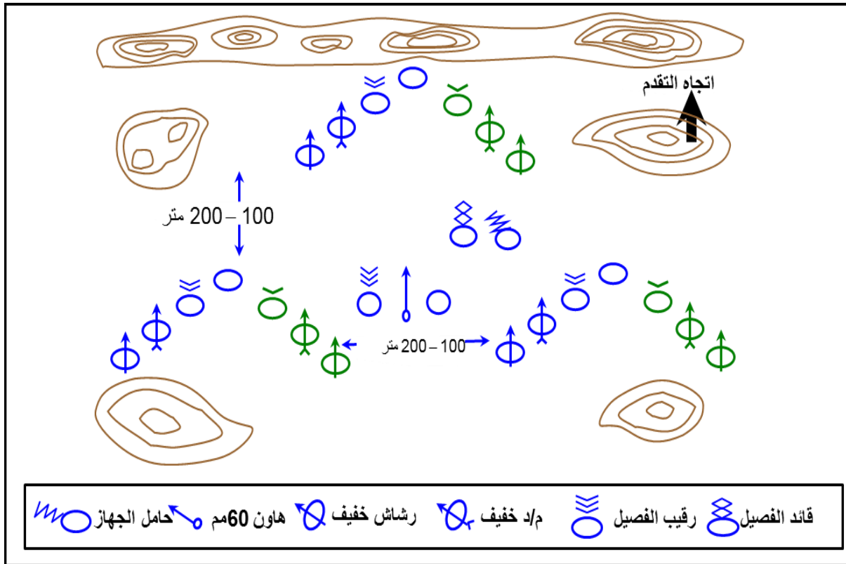
الشكل رقم (47) الحركة كاملة للفصيل
