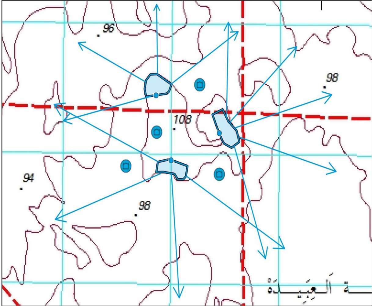
الشكل رقم (16) الدفاع الدائري للفصيل
