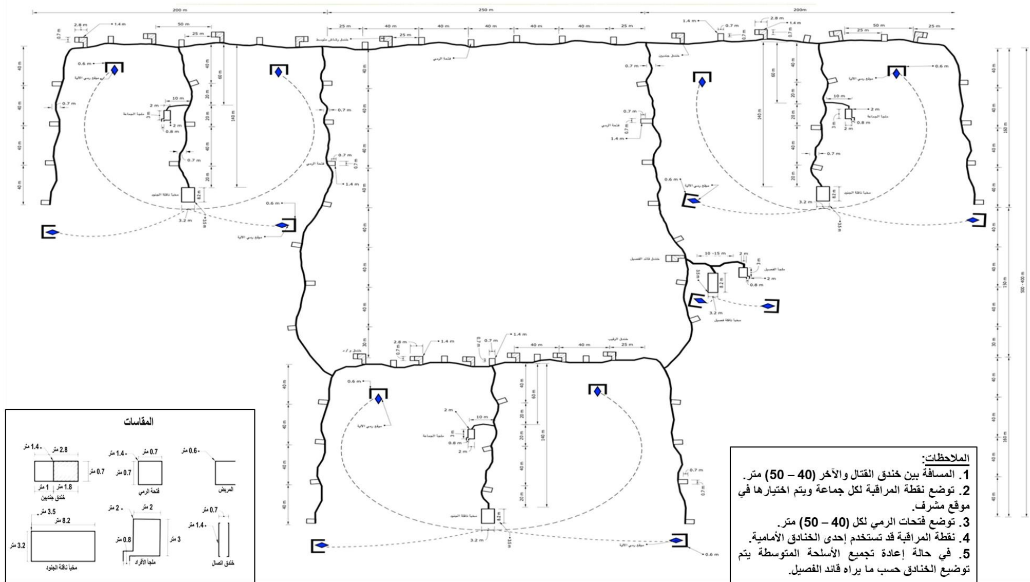
الشكل رقم (22) مثال على موقع دفاعي لفصيل مشاة آلي
