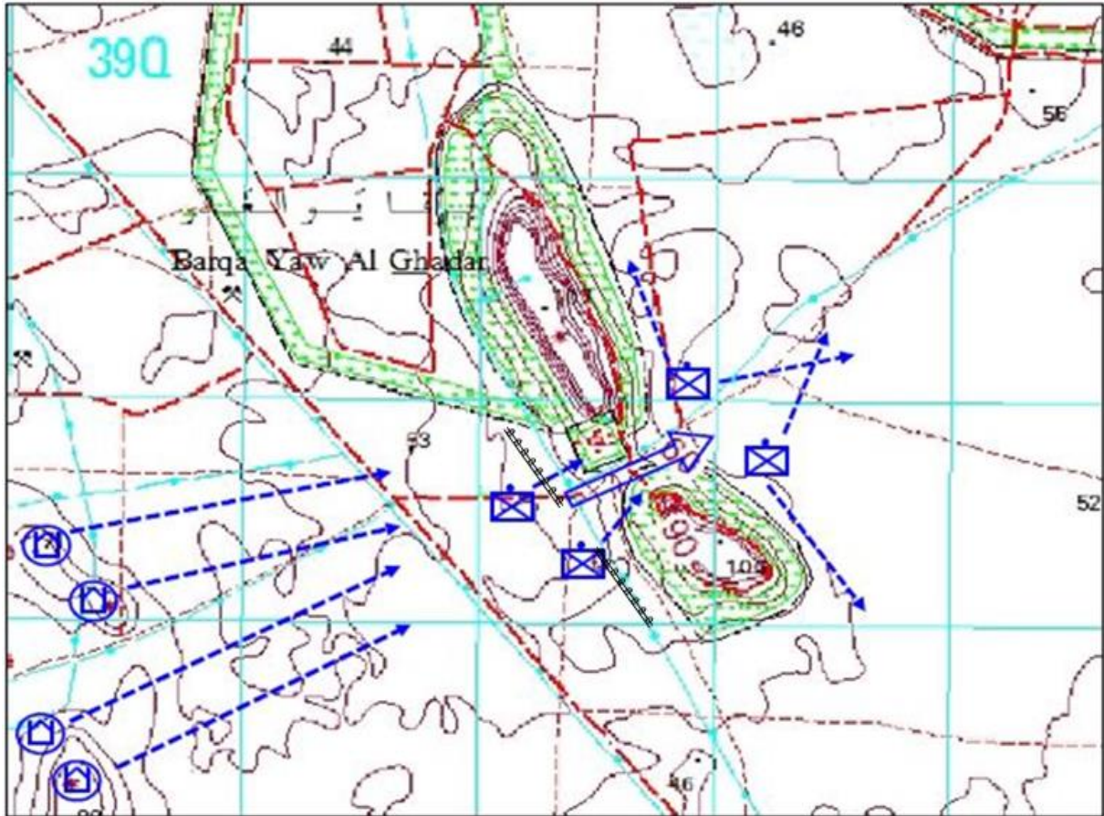
الشكل رقم (64- ج) مراحل اجتياز المانع
