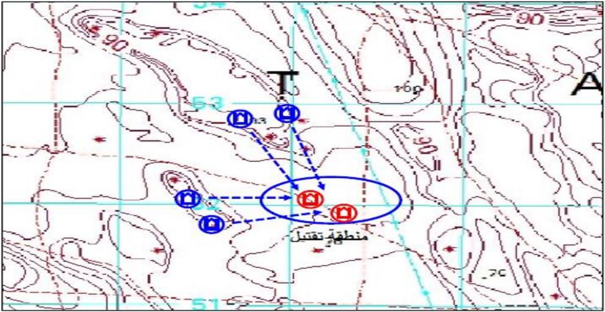
الشكل رقم (69) كمين الفصيل على شكل زاوية
