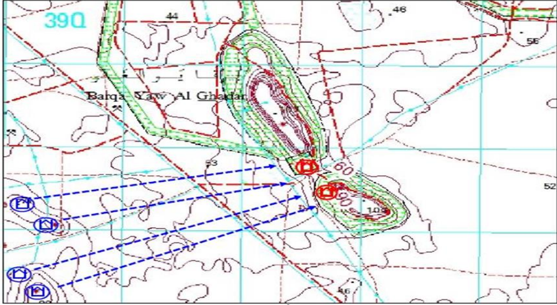
الشكل رقم (64- أ) مراحل اجتياز المانع
