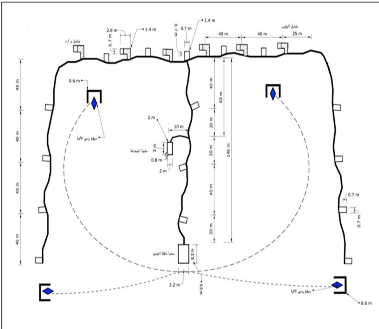
الشكل رقم (21) مثال على موقع دفاعي لجماعة العمق
