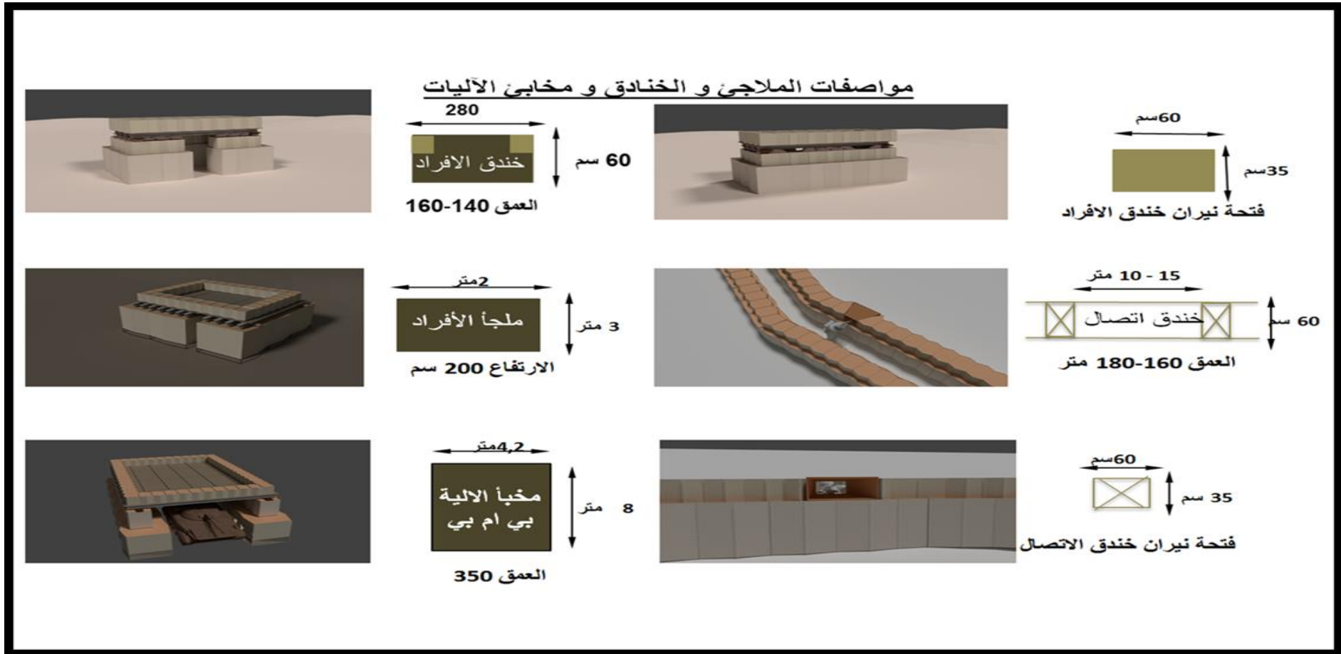
الشكل رقم (35) مواصفات الملاجئ والخنادق ومخابئ الآليات
