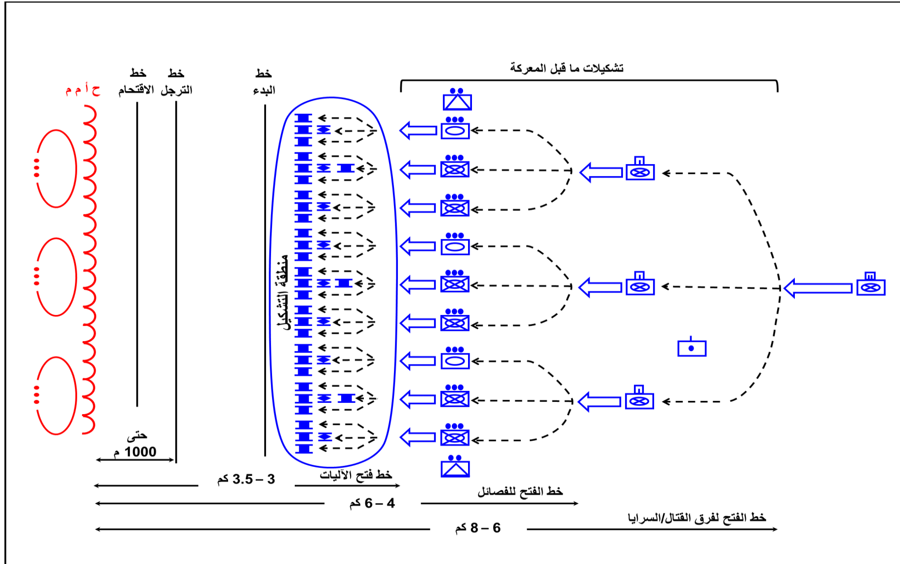
الشكل رقم (66) مثال على خطوط الفتح التعبوي
