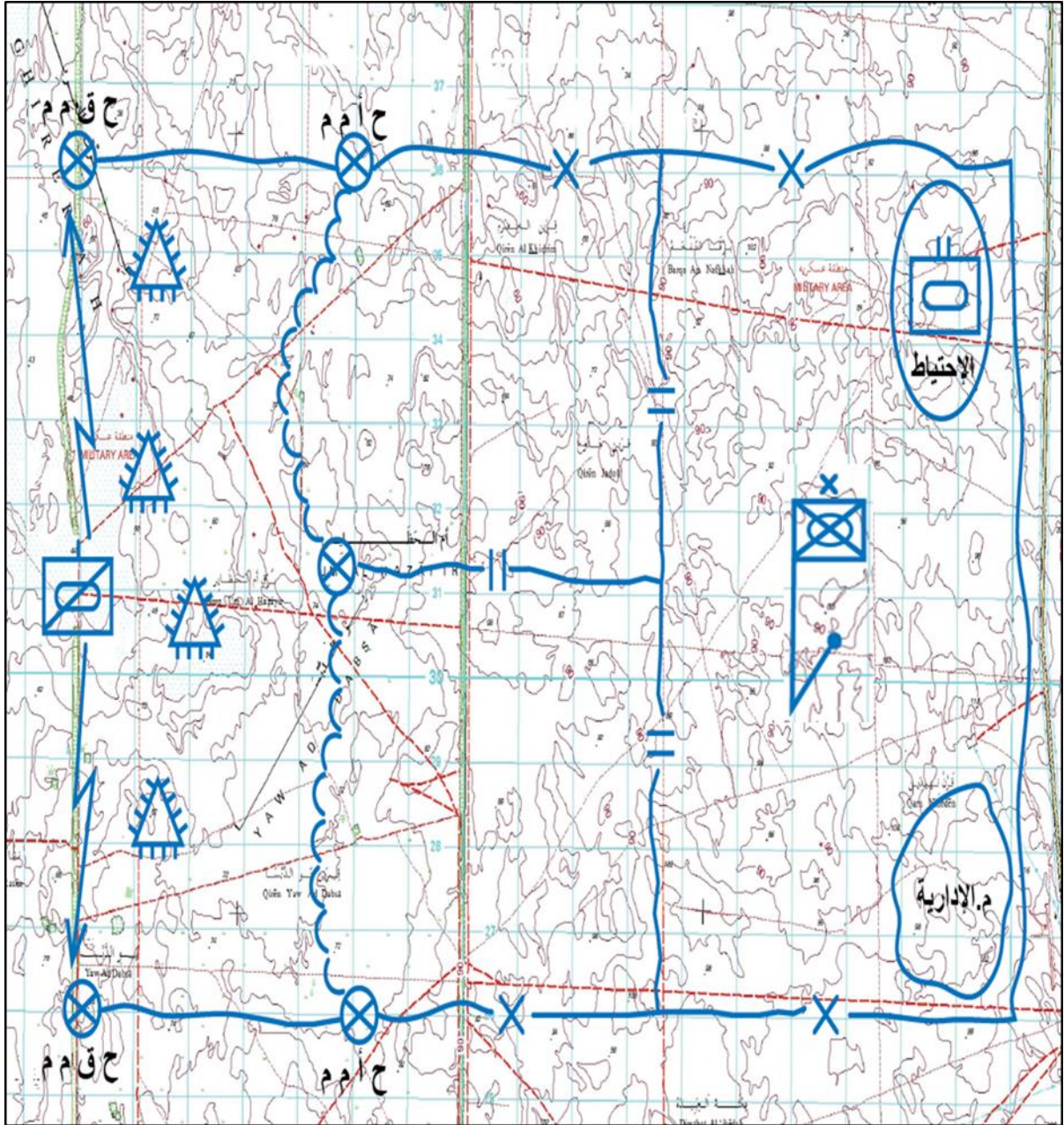
الشكل رقم (19) نقاط قتال خارجية أمام ح أ م م
