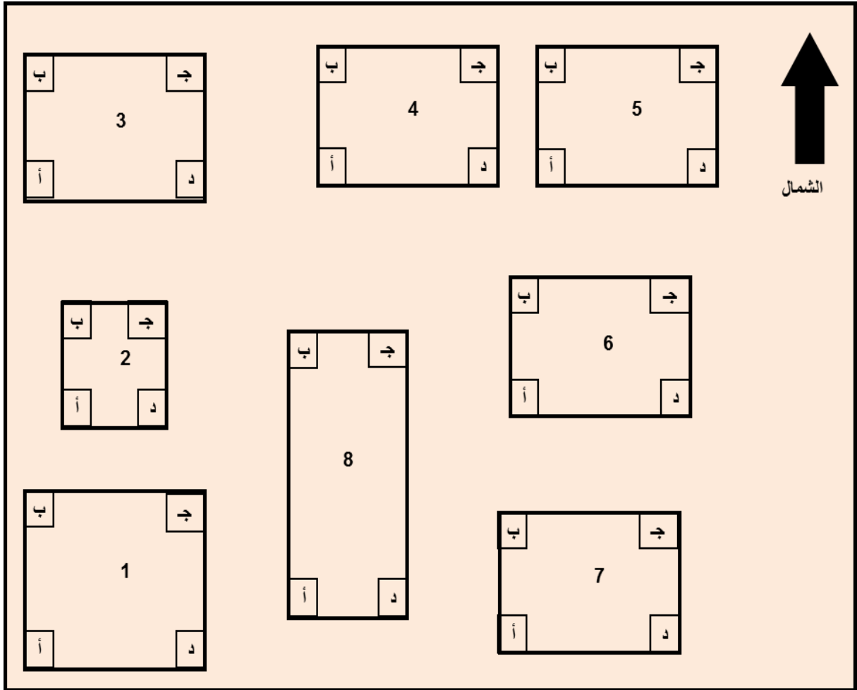
الشكل رقم (3) مثال على نظام ترقيم نقاط مرجع الأهداف في منطقة مبنية
